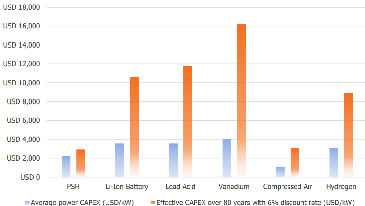
Figura 1 - Comparația costurilor efective pe durata de viață ale tehnologiilor de stocare a energiei pe o perioadă de 80 de ani, (durată de 10 ore, 2020)
