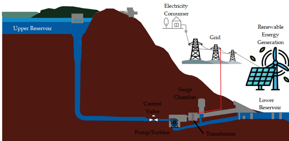
Figura 2 - Un posibil aspect al unui sistem PHES
