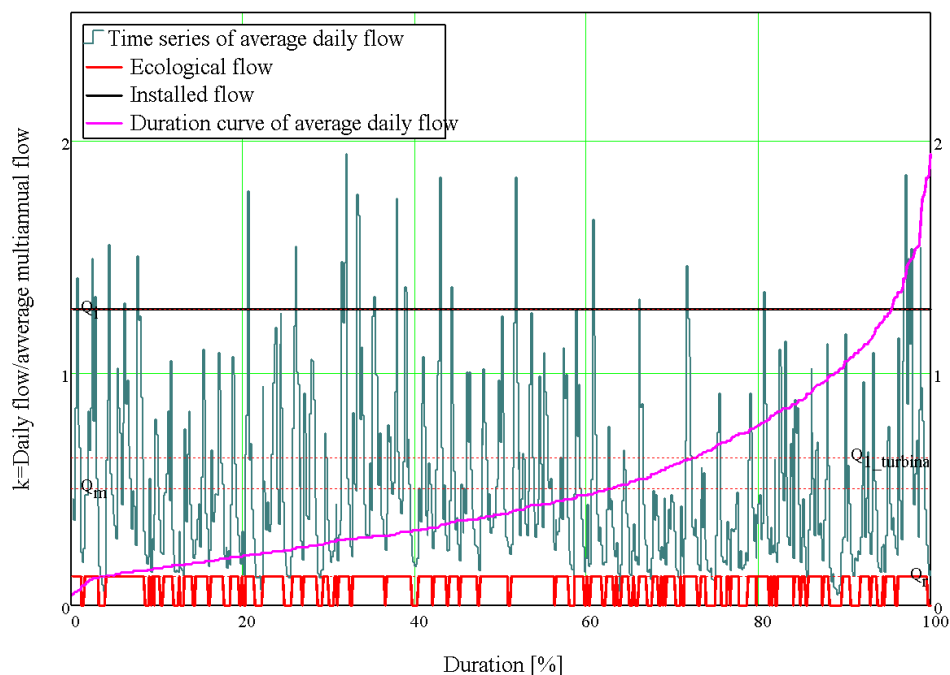
Figura 12. Curba de durată a debitelor medii zilnice.
