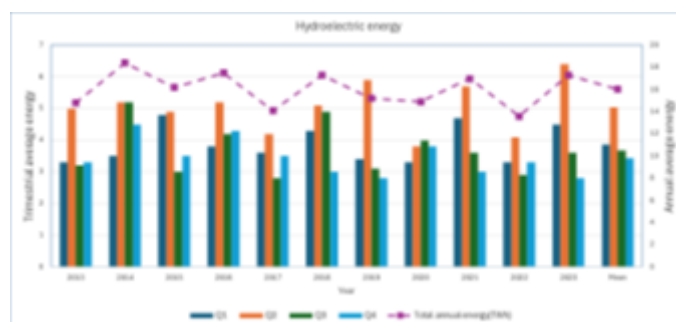
Figura 4. Energia medie trimestrială pentru ultimii 10 ani [12].
